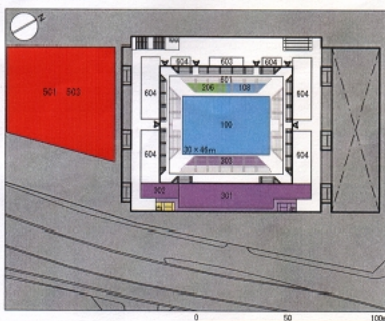
■2階平面図
