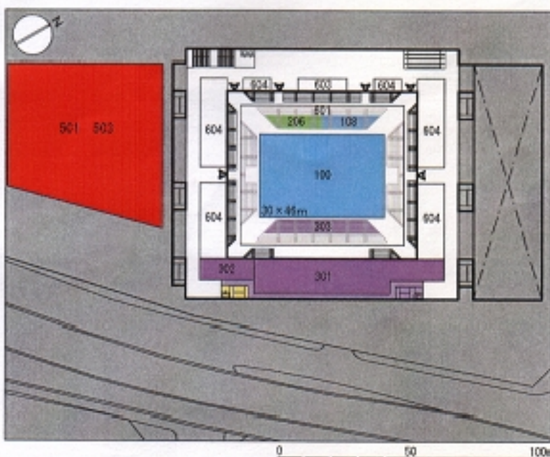
■2階平面図
