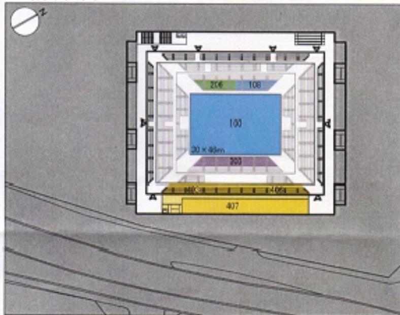
■3階平面図
